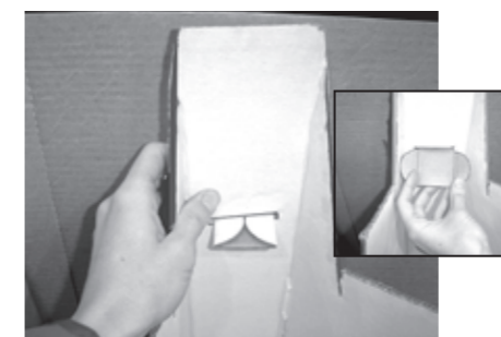
19. Estructuras estantes Encastrarlas en el respaldo, introduciendo las pestañas en las ranuras de la estructura y trabar abriendo las solapas
